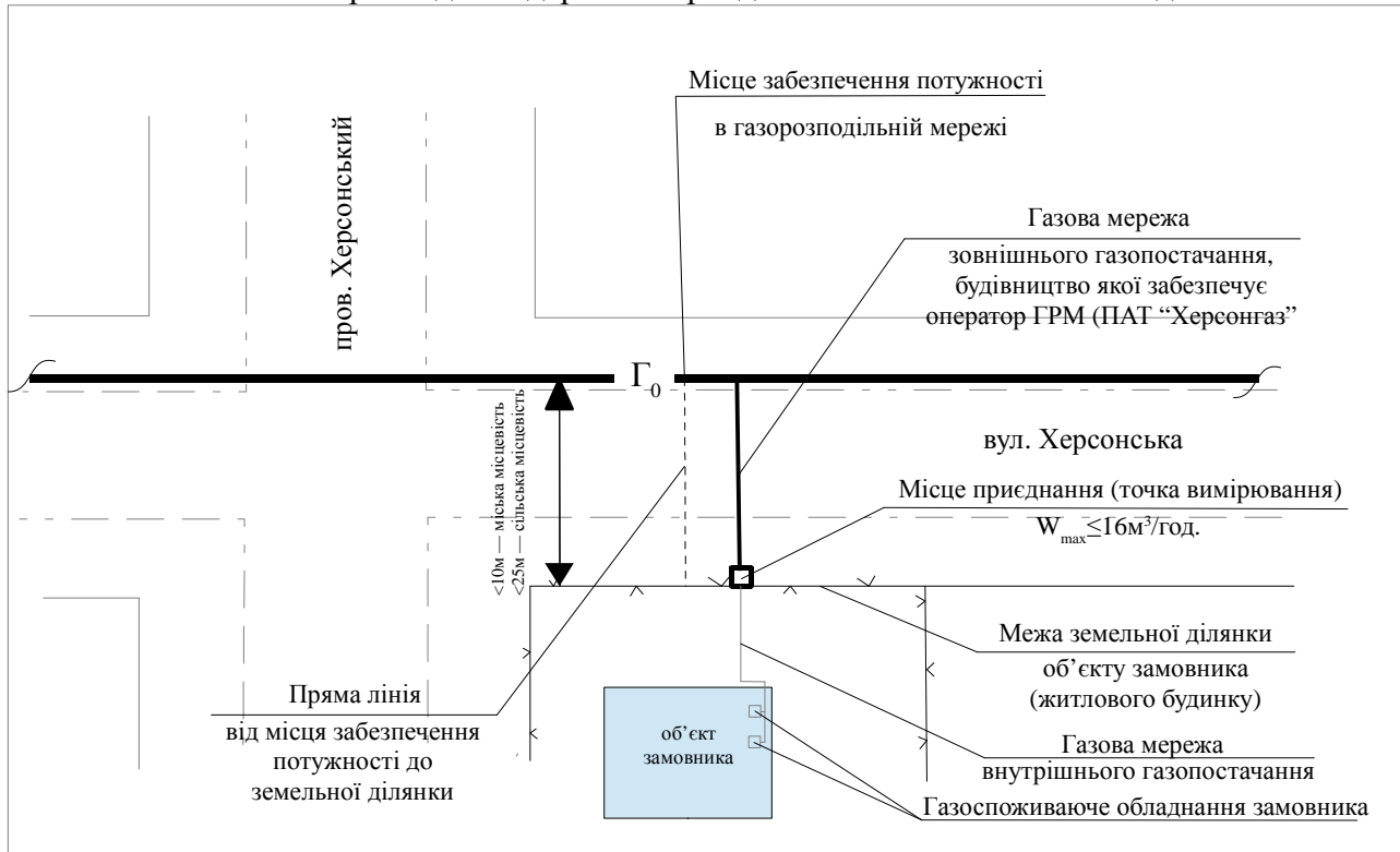
Схема № 1. Приклад стандартного приєднання об'єктів замовників до ГРМ
